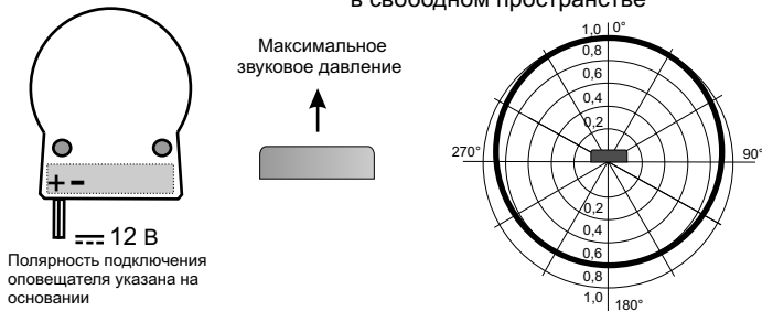
Рис.2 Схема подключения и диаграмма направленности оповещателя ПКИ-МЦ.
