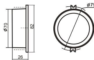
Рис.1. Габаритные и установочные размеры
