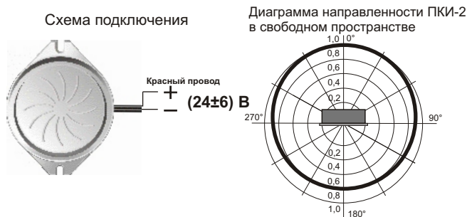
Рис.2 Схема подключения и диаграмма направленности оповещателя ПКИ-2Г.
