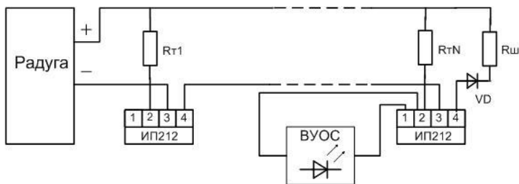
Рисунок А.5 Схема подключения извещателей к прибору «Радуга»
