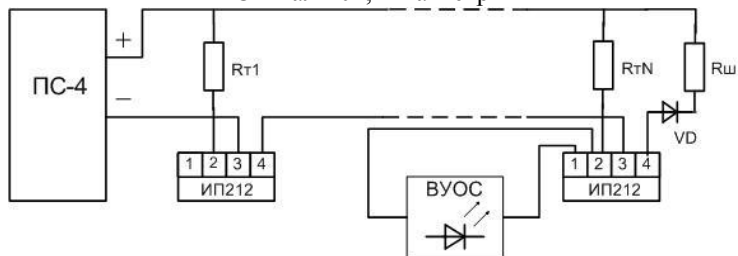
Рисунок А.2 Схема подключения извещателей к приборам «Сигнал-20», «Магистр-2»
