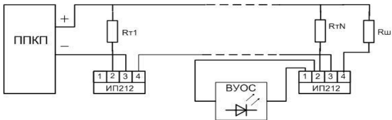
Рисунок А.1 Схема подключения извещателей к приборам ВЭРС-ПК
