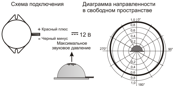
Рис.2 Схема подключения и диаграмма направленности оповещателя ПКИ-МБ.
