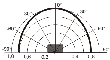
Рис.2 Схема подключения и диаграмма направленности звука оповещателя.
