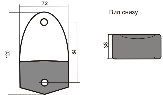
Рис.1. Габаритные и установочные размеры оповещателя
