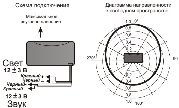
Рис.2 Схема подключения и диаграмма направленности звука оповещателя.
